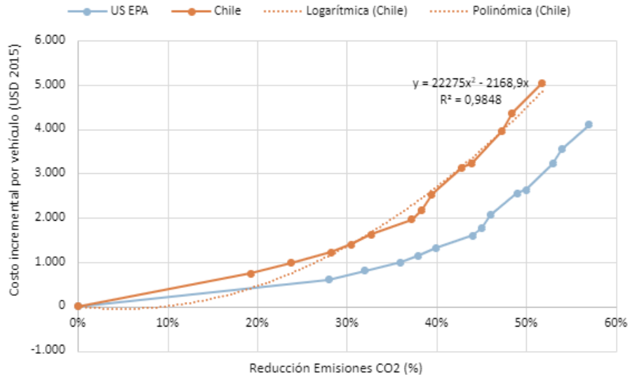
Figura 31 Costo adicional de mejora tecnológica asociado a porcentajes de esfuerzo de reducción de emisiones para camionetas.
