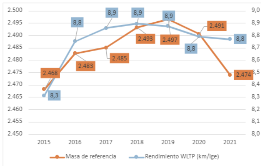
Figura 18 Evolución de indicadores de masa de vehículos y rendimiento energético de vehículos medianos nuevos vendidos en territorio nacional. Periodo 2015 -2021
