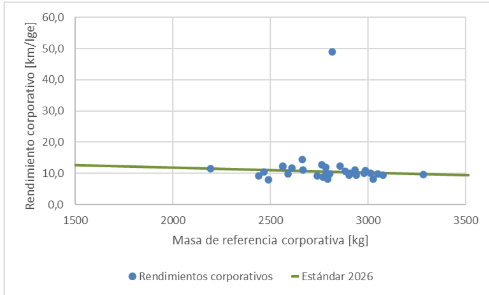
Figura 25 Estándar de rendimiento evaluados y proyectado al año 2026.
