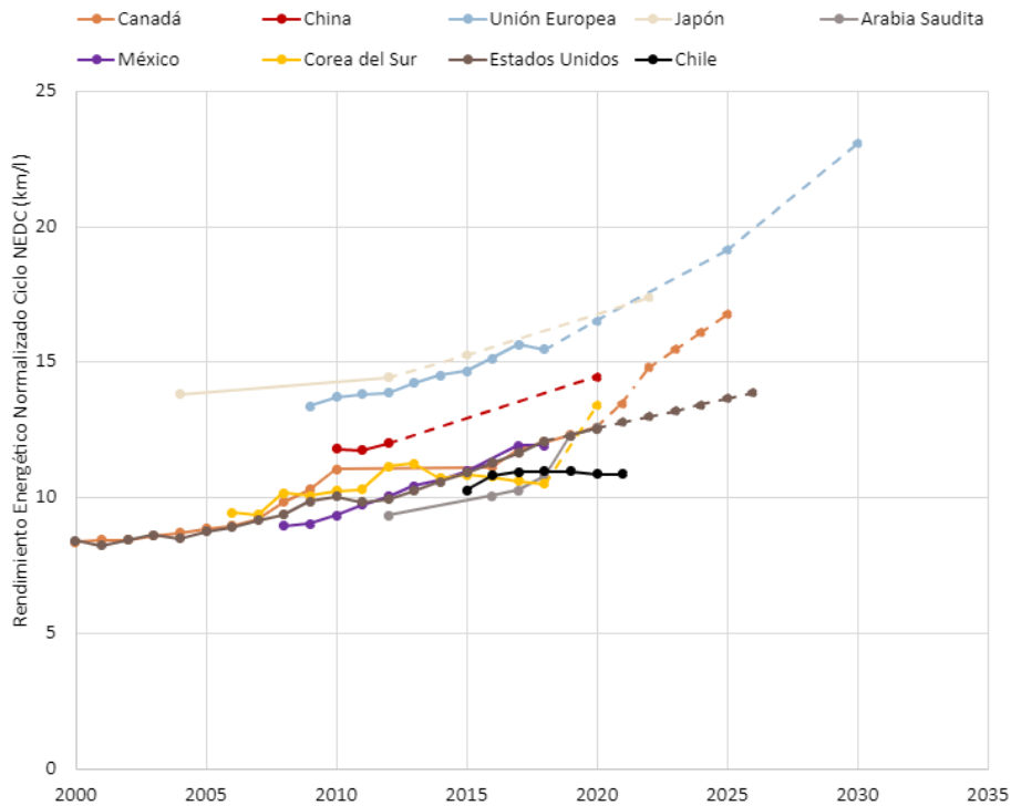
Figura 20: Rendimientos de combustible (en km/l) de vehículos comerciales ligeros nuevos normalizado en ciclo NEDC Fuente: Ministerio de Energía en colaboración con ISCI. Datos (ICCT, 2020)
