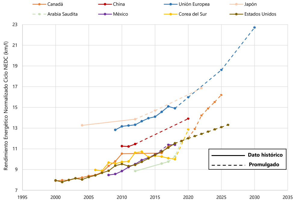
Figura 5 Rendimientos de combustible (en km/l) de vehículos comerciales ligeros nuevos normalizado en ciclo NEDC. Fuente: Elaboración propia. Datos: (ICCT, 2020).
