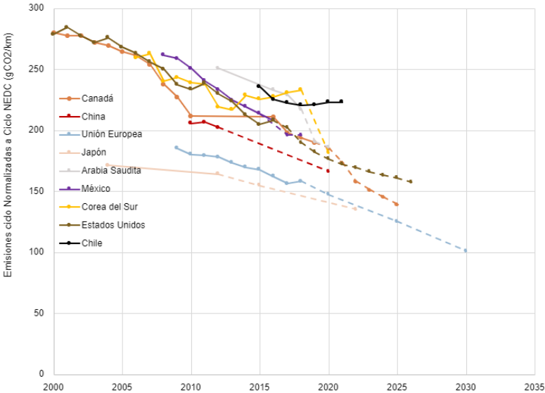
Figura 19 Emisiones (en gCO 2 /km) de vehículos comerciales ligeros nuevos normalizado en ciclo NEDC. Fuente: Ministerio de Energía en colaboración con ISCI. Datos (ICCT, 2020).
