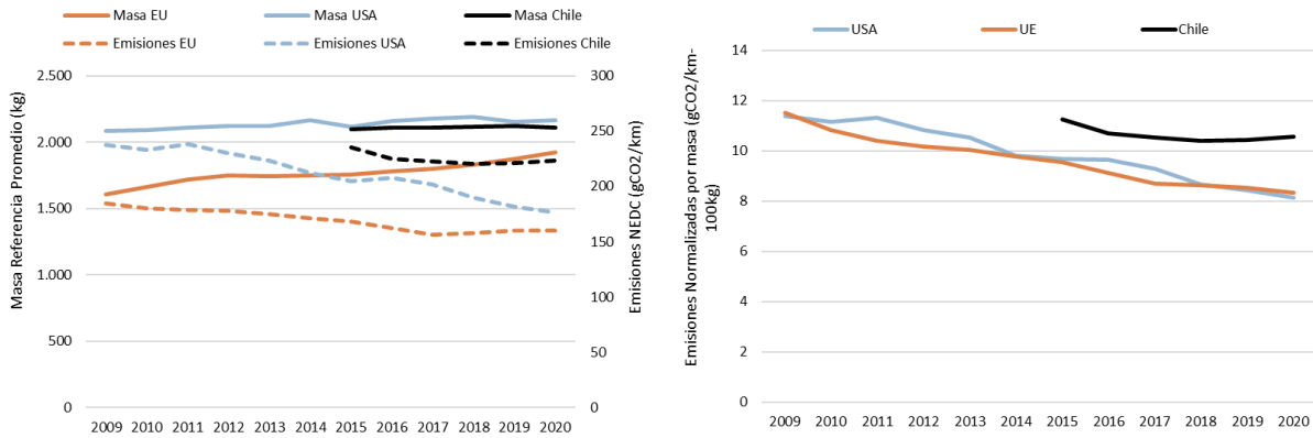
Figura 21 Comportamientos históricos de masa promedio y emisiones promedio del mercado de vehículos medianos Chile, USA & EU.
