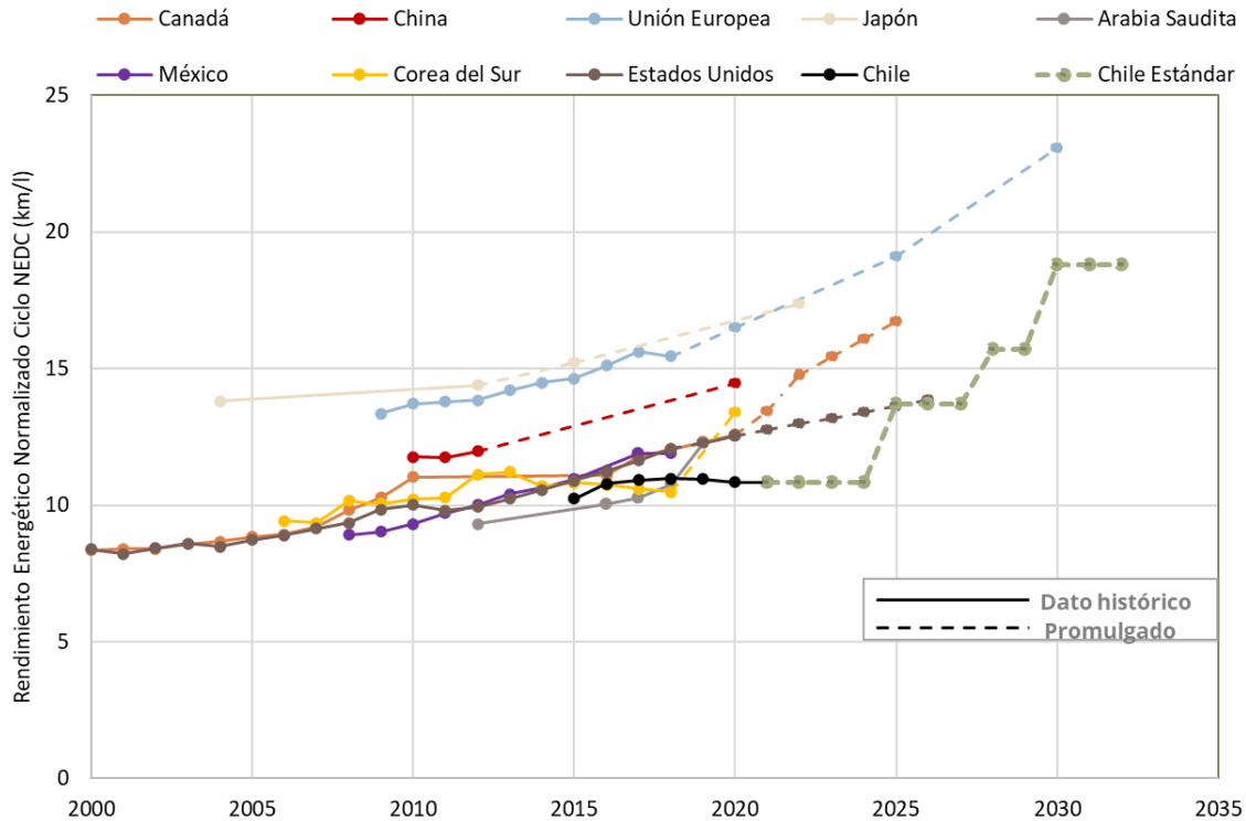
Figura 23 Propuesta estándar de rendimiento para vehículos medianos en el contexto internacional y nacional normalizados al ciclo NEDC.
