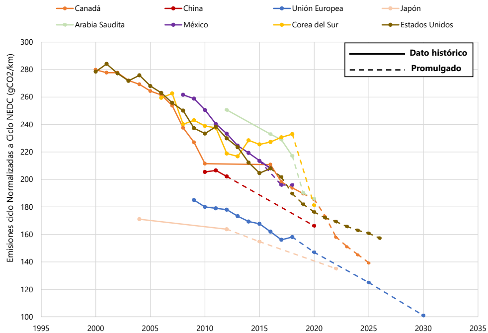
Figura 6 Emisiones (en gCO2/km) de vehículos comerciales ligeros nuevos normalizado en ciclo NEDC. Fuente: Elaboración propia. Datos: (ICCT, 2020).
