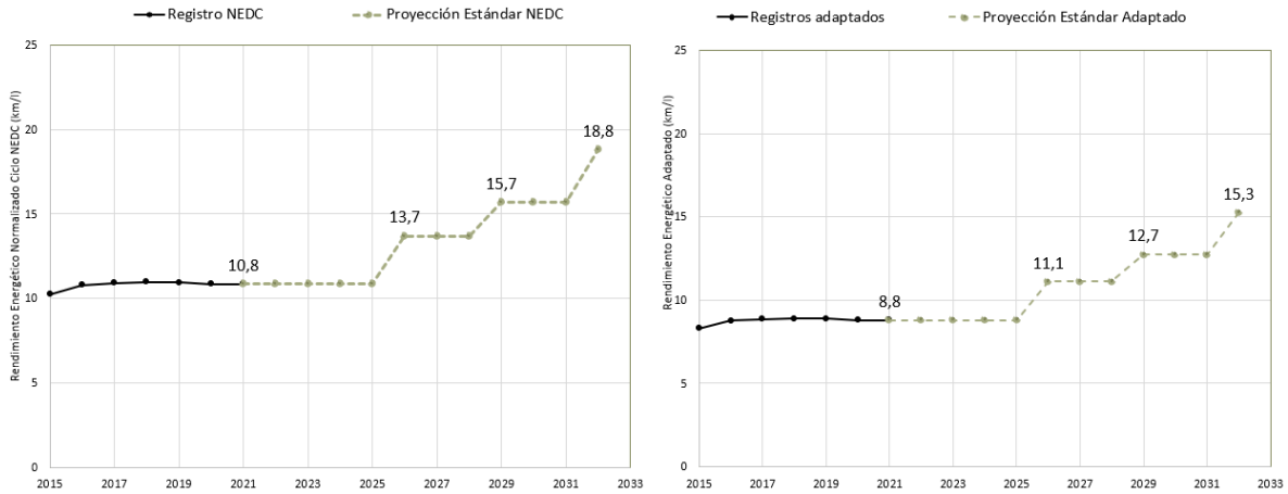
Figura 24. Propuesta de estándar de rendimiento para vehículos medianos en ciclo NEDC (izquierda) y ciclo NEDC adaptado (derecha).
