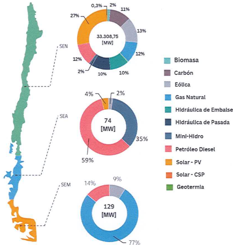
Figura 2: Composición de la capacidad instalada de generación eléctrica (SEN) a julio de 2024.
