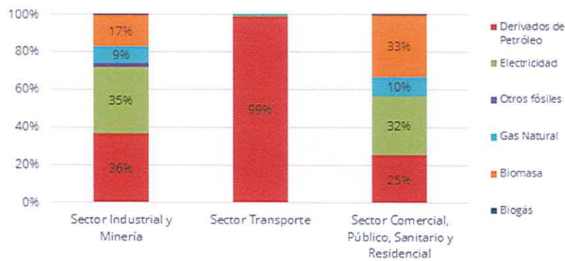
Figura 1: Participación de energéticos en los principales sectores de consumo final, año 2022.
