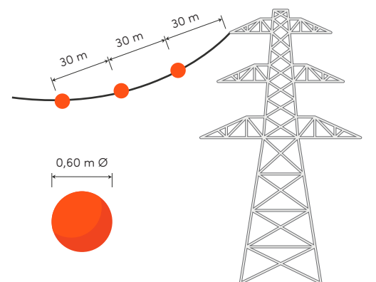
Señalización de la línea eléctrica
