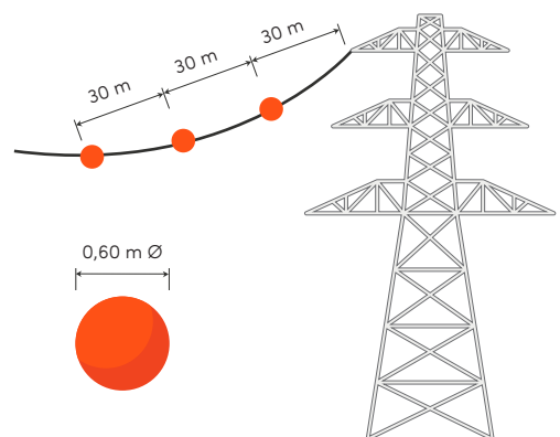
Señalización de la línea eléctrica
