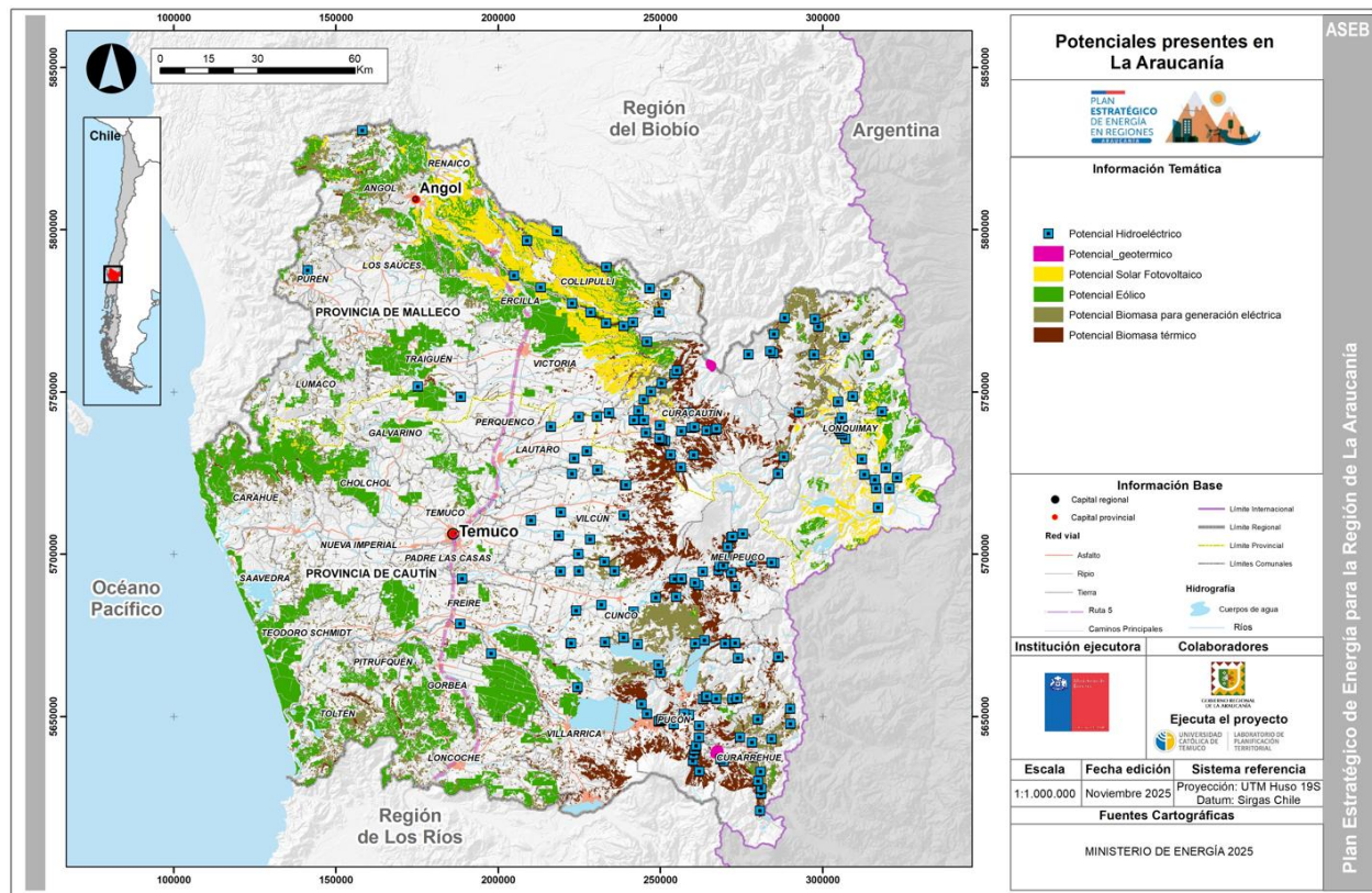
Figura 11 Espacialización de los potenciales energéticos presentes en la región de La Araucanía.
