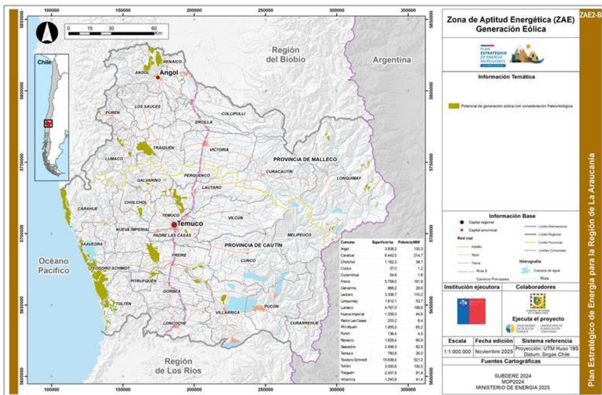
Figura 58 ZAE 2-B Generación eólica con consideración paleontológica
