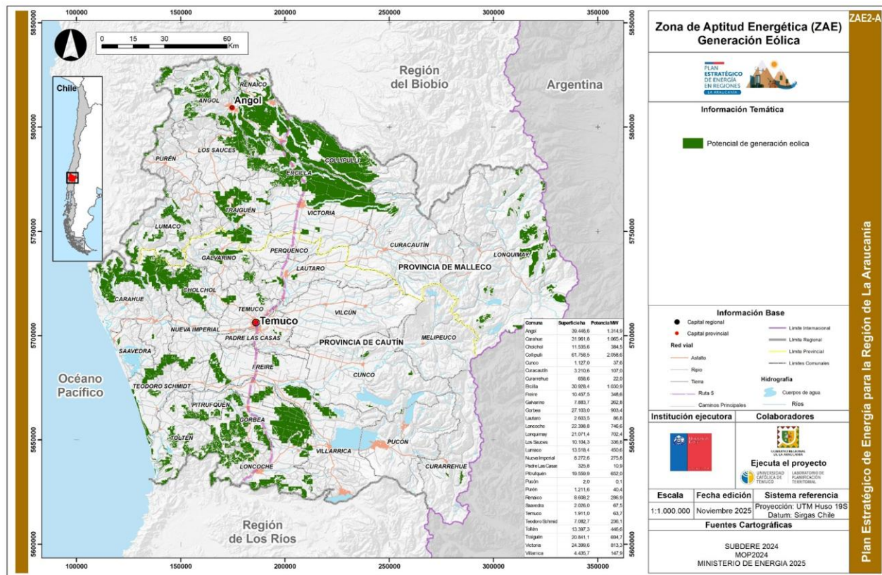
Figura 57 ZAE 2-A Generación eólica
