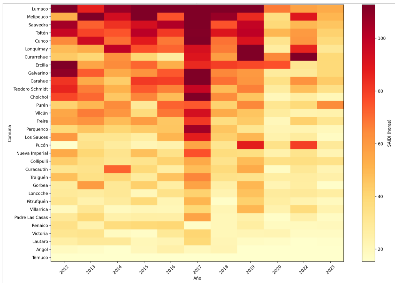
Figura 19 Evolución anual de SAIDI comunal (2012-2023) de la región de La Araucanía.
