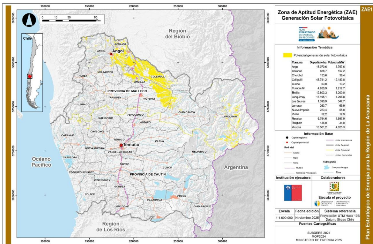
Figura 56 ZAE 1 Generación solar fotovoltaica
