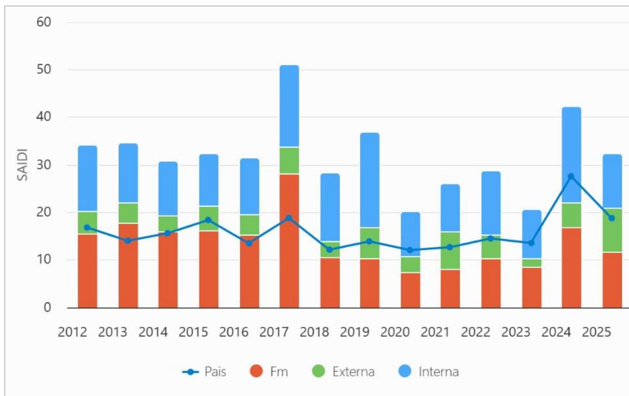
Figura 18 Evolución anual de SAIDI (2012-2025) en la región de La Araucanía
