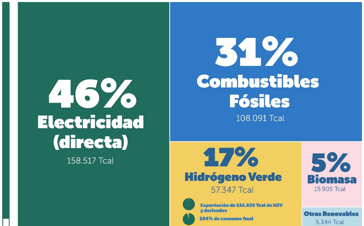
Figura 4: Consumo Final de Energía en Chile, 2050. PELP: Escenario Carbono Neutralidad: 349.959 Tcal.
