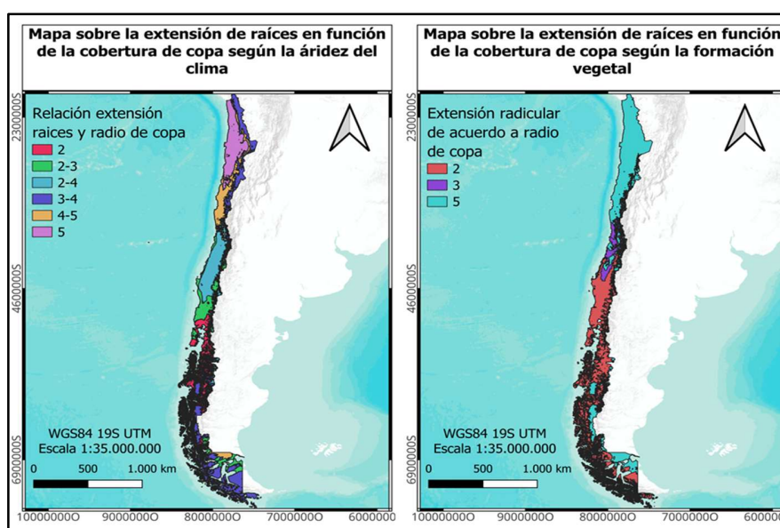
Figura 1. Mapa de la extensión radicular lateral en función del radio de copa según aridez del sistema como sugerencia para la estimación de la extensión radicular en un contexto precautorio y de incertidumbre.
