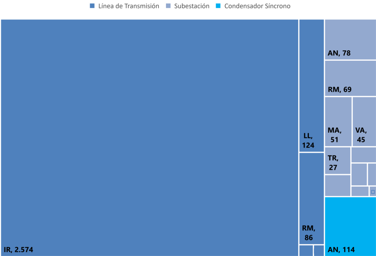
Inversiones en USD millones en obras de transmisión según tipo y región, al 30 de junio de 2026
