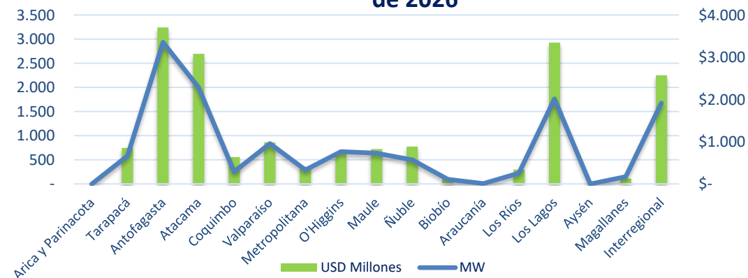
Inversión en USD millones y capacidad en MW de centrales de generación en calificación al 30 de junio de 2026
