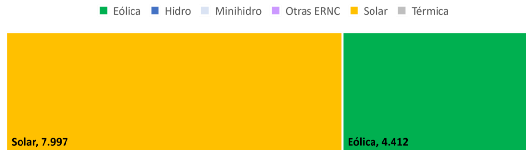
Capacidad de centrales de generación en calificación en el SEIA en MW según tecnología al 30 de junio de 2026
